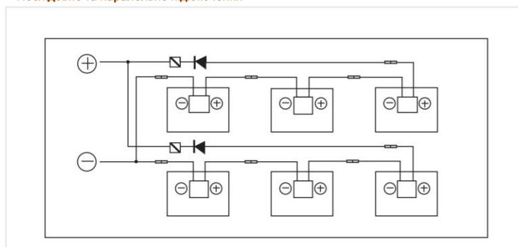
Послідовне та паралельне підключення
